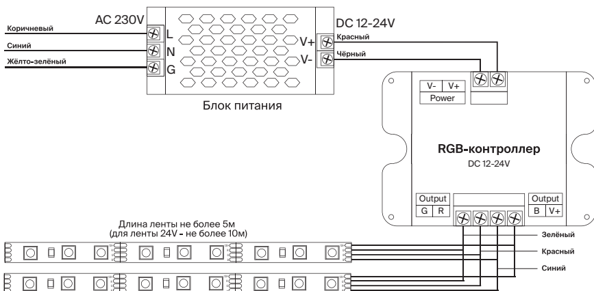
Рис. 1 схема подключения контроллера
